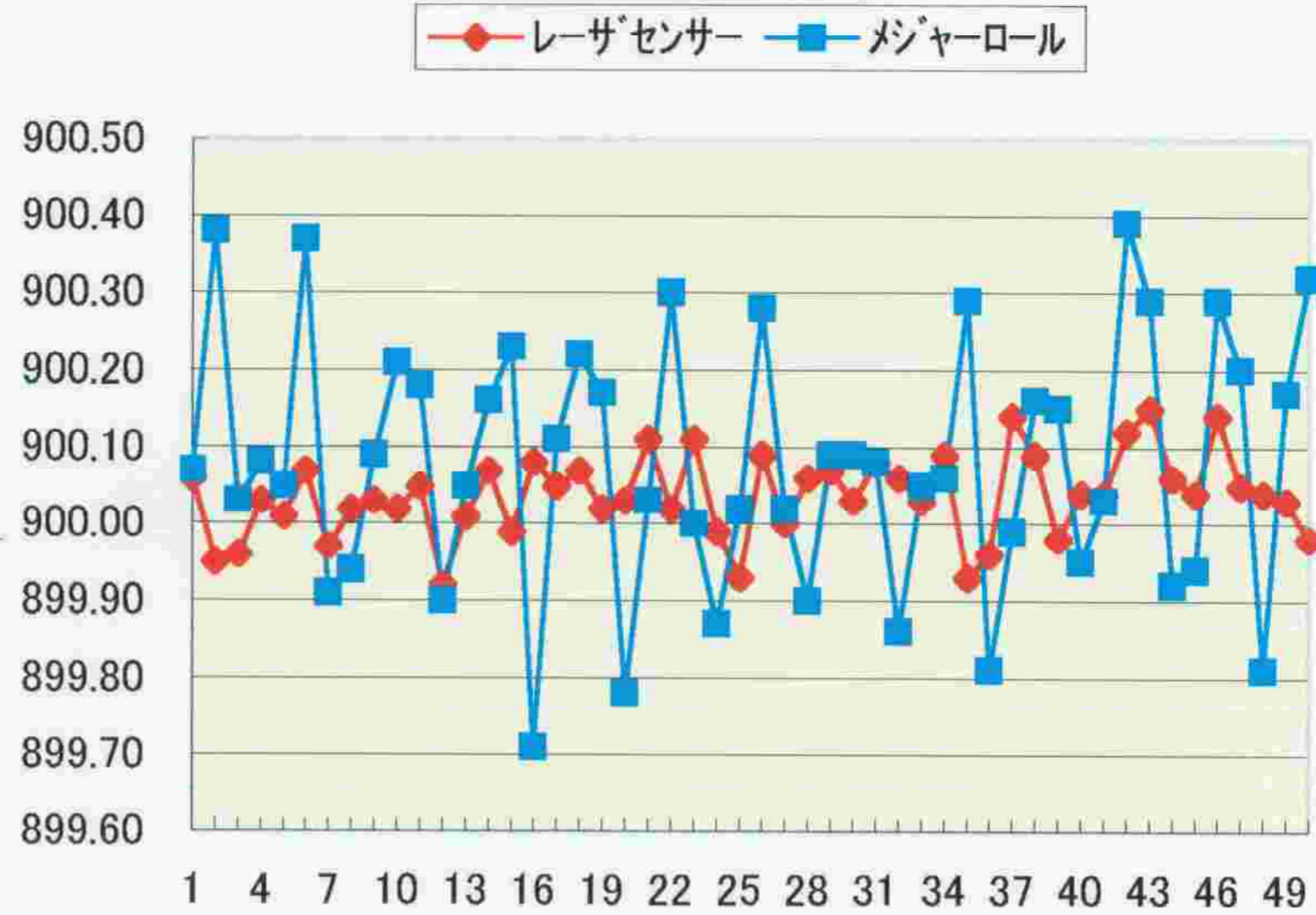
測長データ
